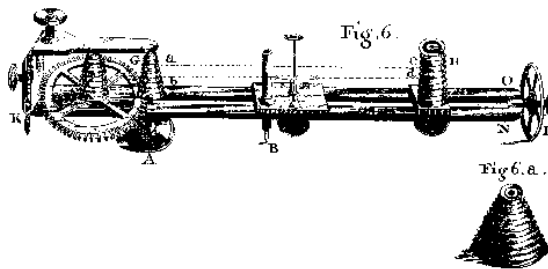
Fig. 60: Heliograph von George Adams (1791)
