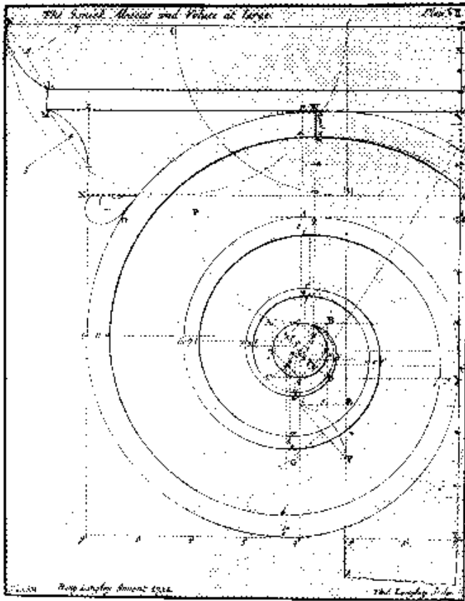
Fig. 62: Spirale ohne Zentrum
