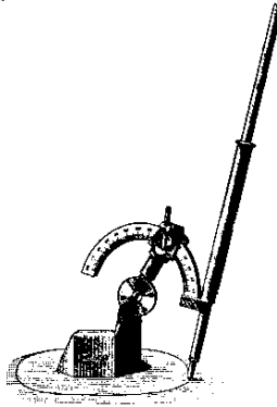
Fig. 56: Zeichenebene als Kegelschnittebene, aus Dyck 1994
