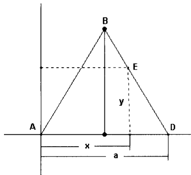
Fig. 46: Ellipsenzeichninstrument nach Frans von Schooten
