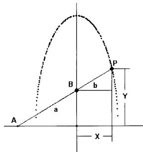
Fig. 50: Mathematische Erklärung
