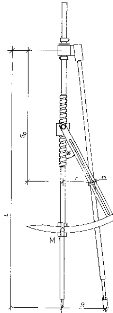
Fig. 65: Konstruktionszeichnung nach Leyerer
