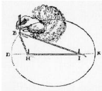
Fig. 41: Fadenkonstruktion der Ellipse nach Descartes, 1637, S.90
