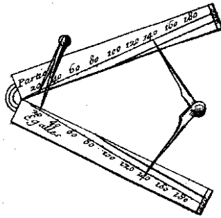
Fig. 36: Prinzip des Proportionalzirkels; N. Bion: Traité de la construction et des principaux usages des instrumens mathématique, Paris 1752
