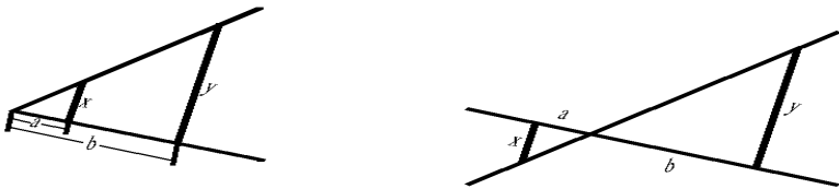
Fig. 35: Strahlensatzfiguren
