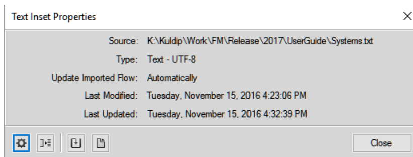
Figure 5: Dialogfeld „Texteingeschubeigenschaften“
