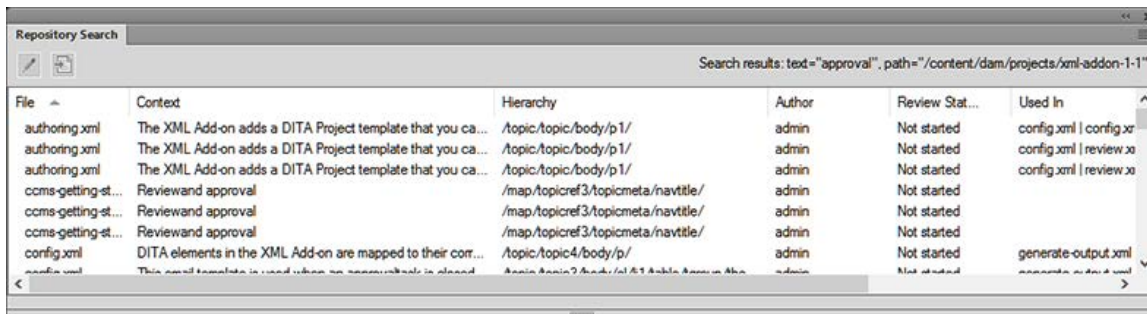
Figure 3: Fenster „Repository-Suche“
