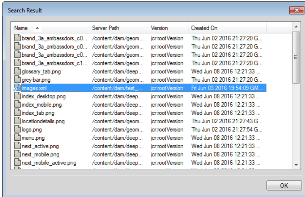
Figure 2: Dialogfeld „Suchergebnis“
