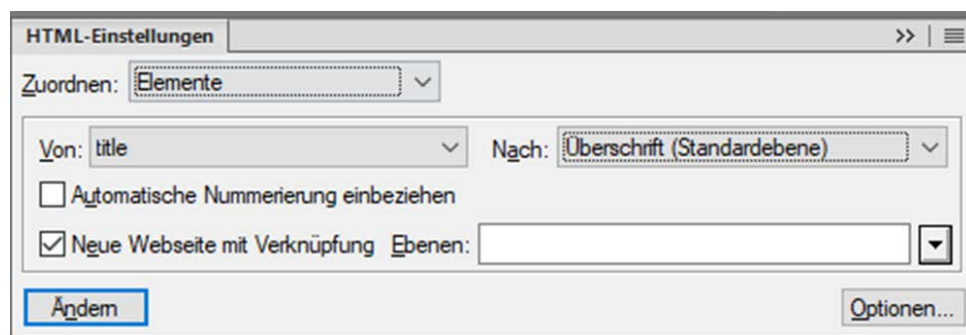
Figure 1: Dialogfeld „HTML-Einstellungen“
