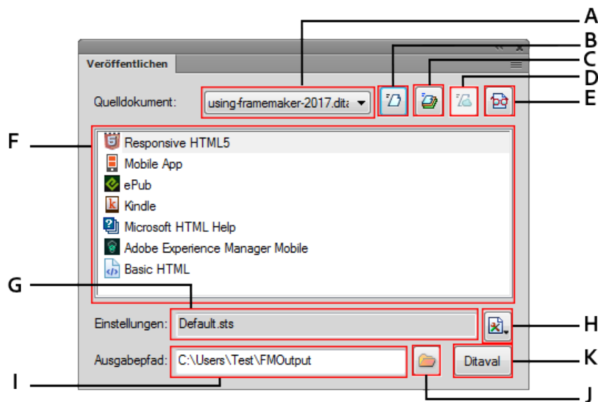
Figure 1: Bedienfeld „Veröffentlichen“
