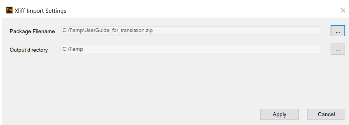
Figure 1: Dialogfeld „XLIFF-Import-Einstellungen“
