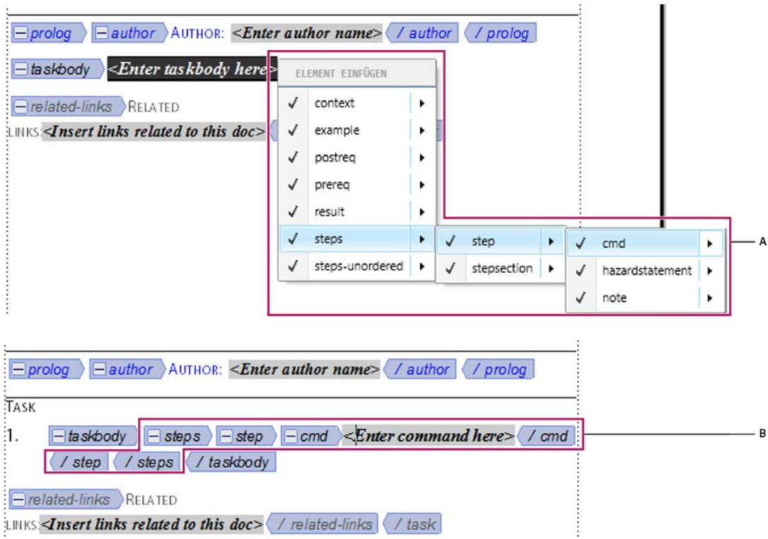
Figure 2: Elementhierarchie einfügen
