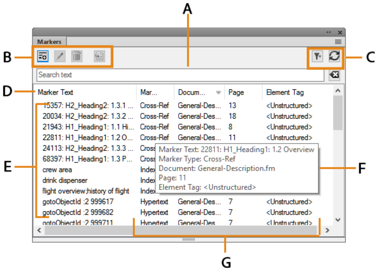
Figure 1: Fensterbenutzeroberfläche
