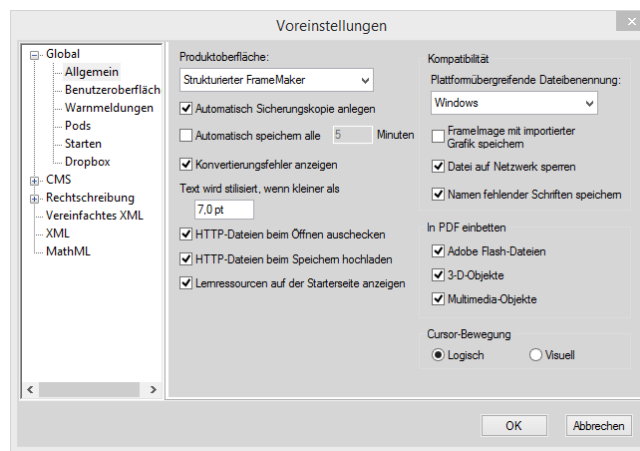
Figure 1: Dialogfeld „FrameMaker-Voreinstellungen“
