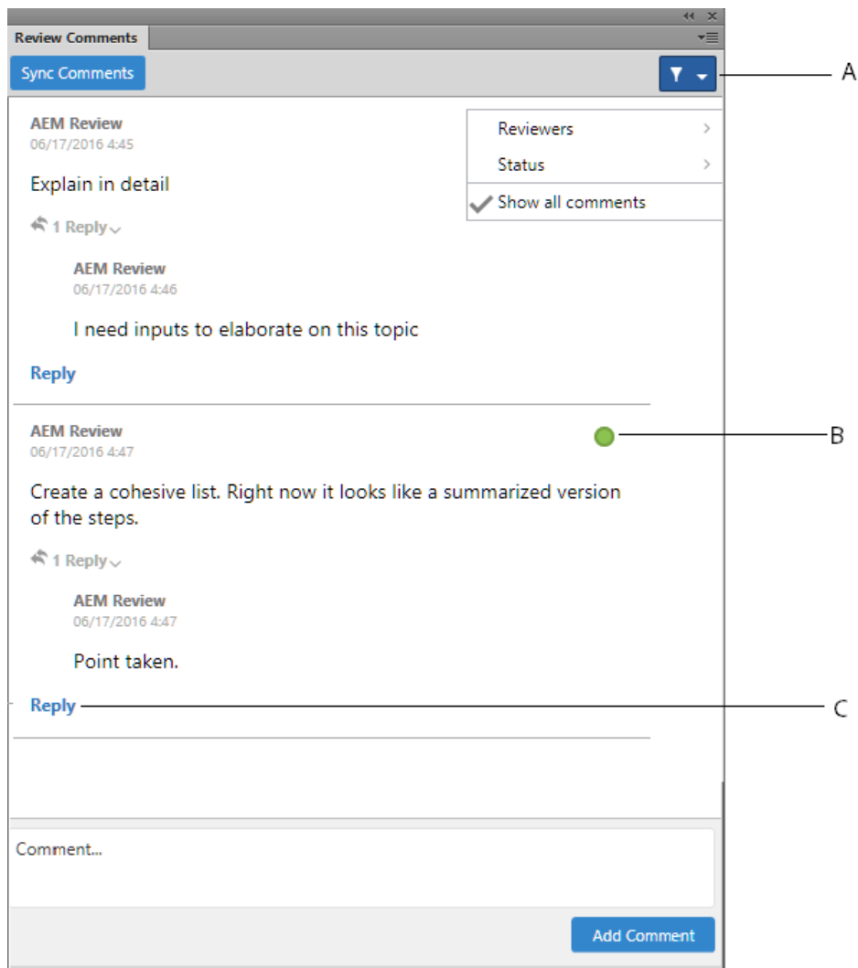
Figure 1: Fenster „Prüfkommentare“
