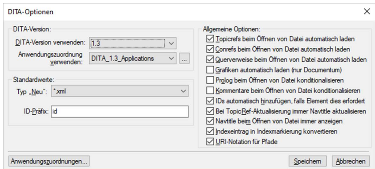
Figure 1: Dialogfeld „DITA-Optionen“
