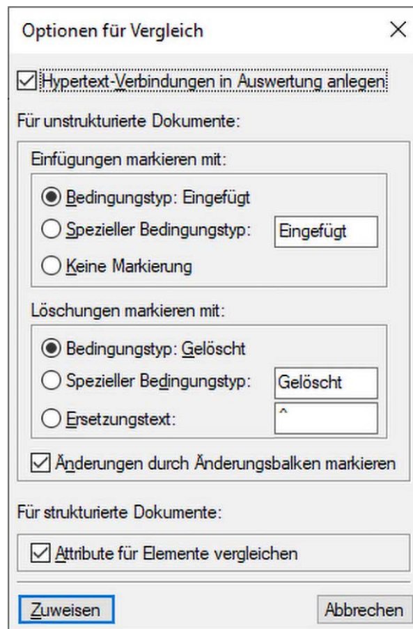
Figure 3: Dialogfeld „Vergleichsoptionen“
