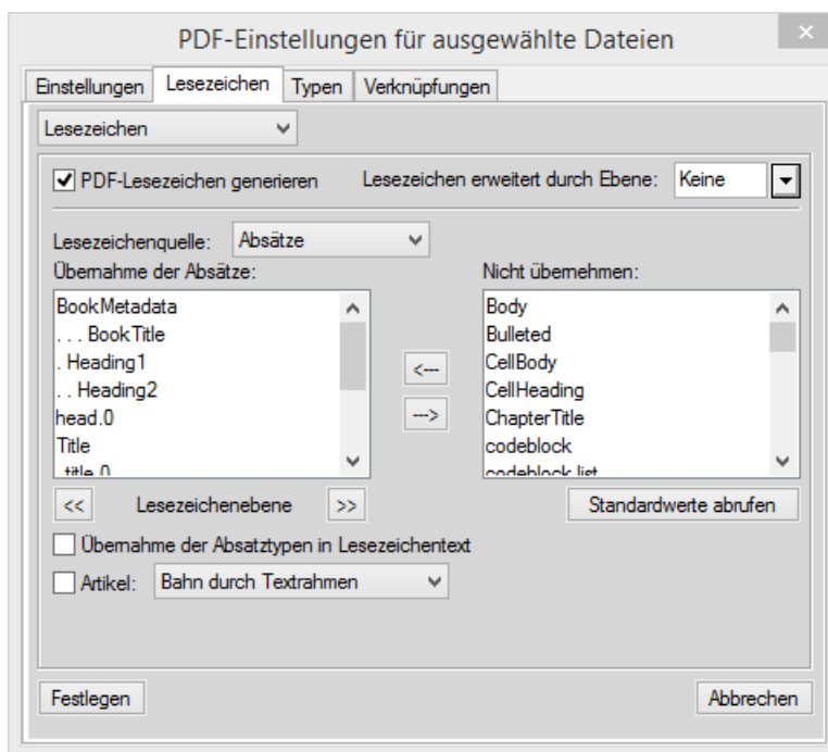
Figure 1: Dialogfeld „PDF-Einstellungen“
