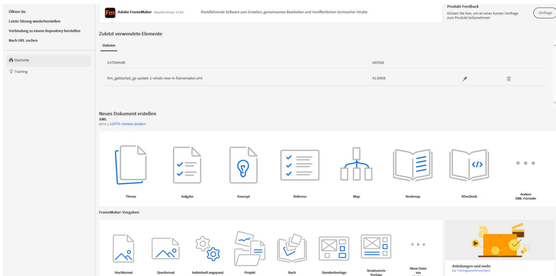
Figure 1: Begrüßungsbildschirm
