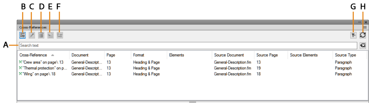
Figure 1: Fenster „Querverweise“
